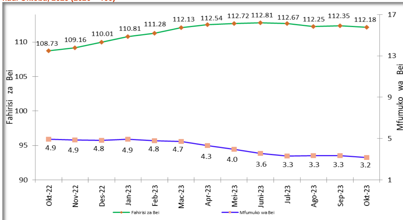
Kielelezo Namba 1: Mwenendo wa Fahirisi za Bei za Taifa na Mfumuko wa Bei Kutoka Mwezi Oktoba, 2022 hadi Oktoba, 2023 (2020 = 100)
