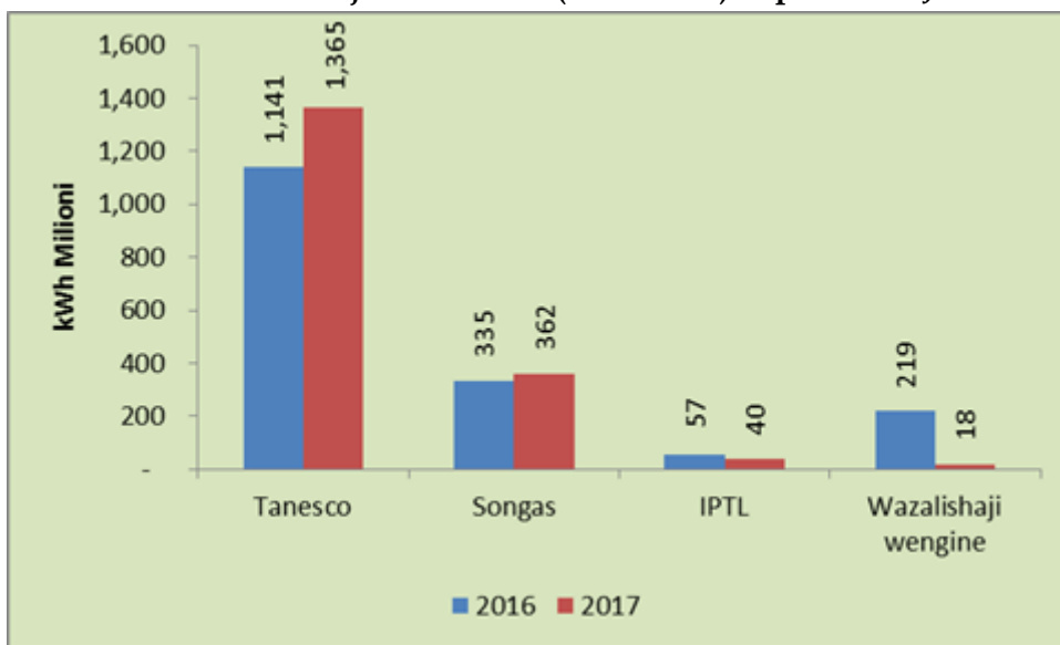
Mchoro Na. 4: Uzalishaji wa Umeme (Mill. Kwh) Kipindi cha Januari - Machi, 2016 - 2017
